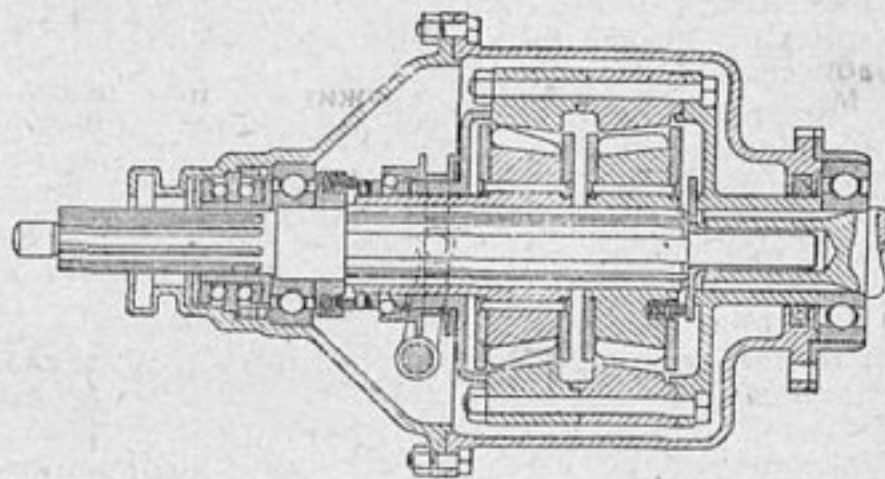
Механизм свободного хода системы „Humfrey Landberg“
